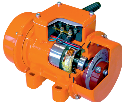
Vibrasyon Motorlar / External Vibration Motor / محرك رجاج
