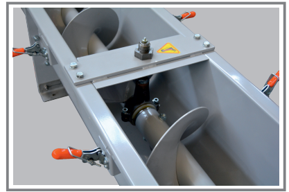
Asma Yatak Hanger Bearing شلال الحلزون الوسطي
