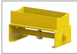
Bakım ve Temizleme Kapağı Cleaning and Maintenance Cover غطاء الصيانة والتنظيف
