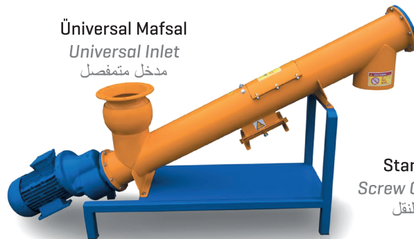
Çimento Helezonu Cement Screw Conveyor حلزون نقل الإسمنت
