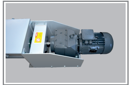
R. Motor Bağlantı R. Motor Mounting تركيب المحرك
